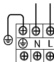
Terminal de conexión tensión alimentación
