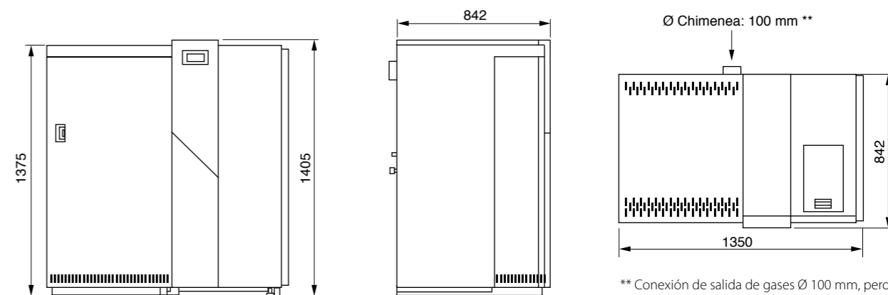
DIMENSIONES DE BIOMASTER 25 Y 32 CON TOLVA DE 230 KG
