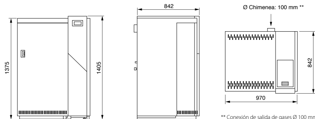
DIMENSIONES DE BIOMASTER 25 Y 32 CON TOLVA DE 112 KG
