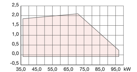
CURVA DE FUNCIONAMIENTO Quemador BENTONE B2-S de bajo NOx
