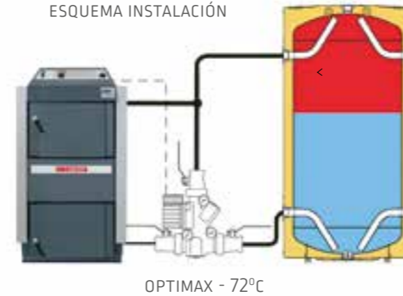
ESQUEMA INSTALACIÓN
